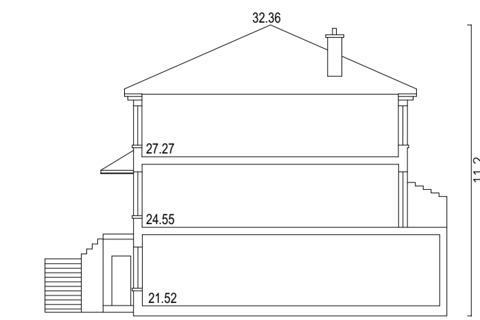
Datum 15.00 AOD Section A-A
